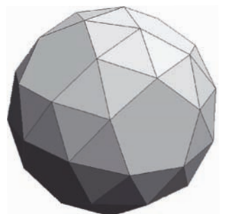
変形12面体という多面体です
